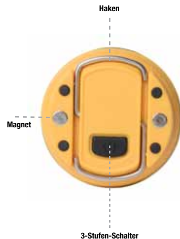
3-Stufen-Schalter
